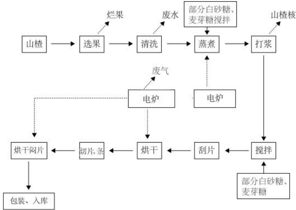
图 1 工艺流程及产污环节示意图
