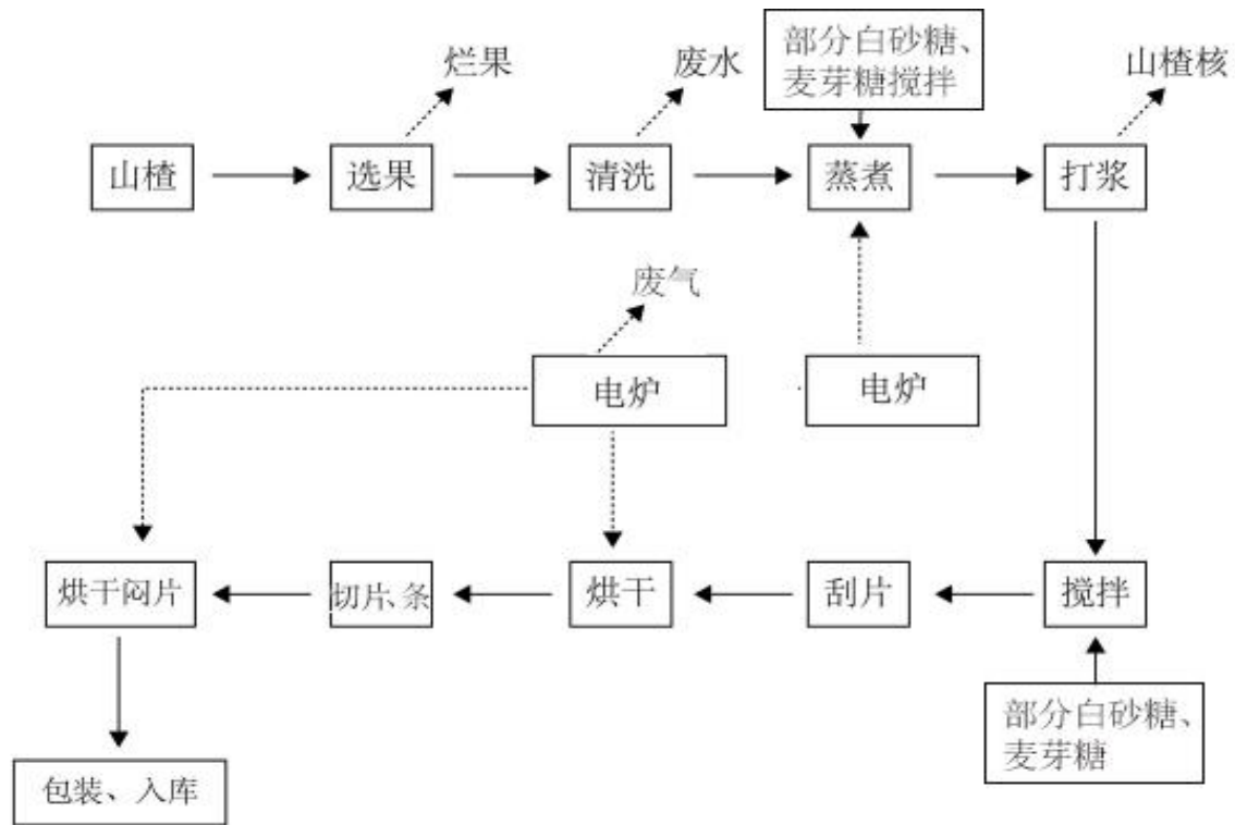
图 2.3-1 工艺流程及产污环节示意图
