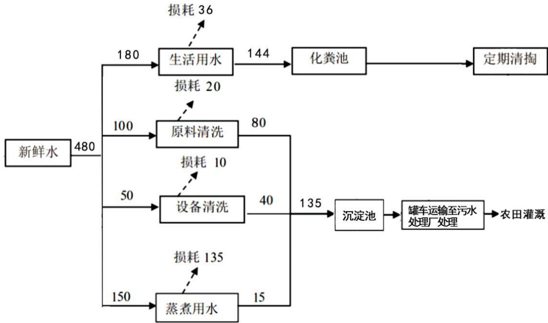
图 2.2-2 项目水量平衡图 单位：m³/a
