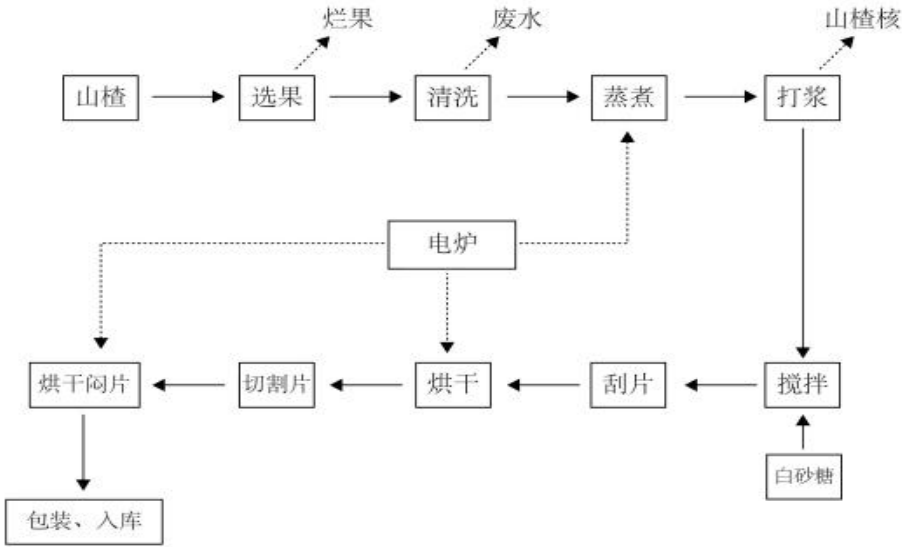
图 2.3-1 工艺流程及产污环节示意图
