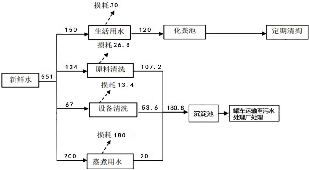
图 2.2-2 项目水量平衡图 单位：m 3 /a
