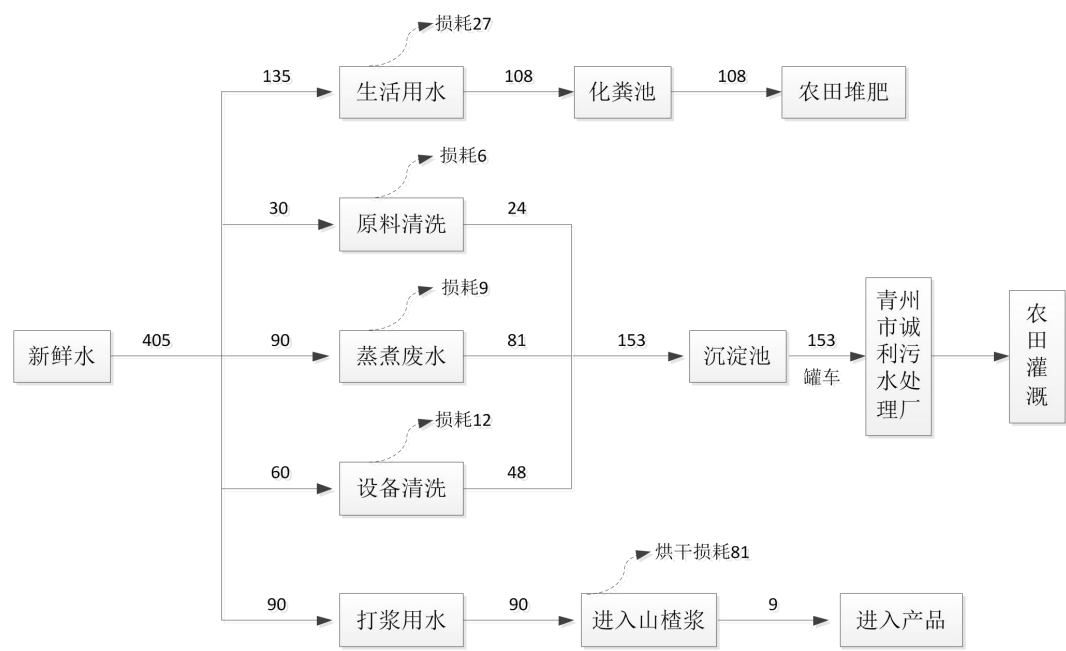
本项目水量平衡图：
