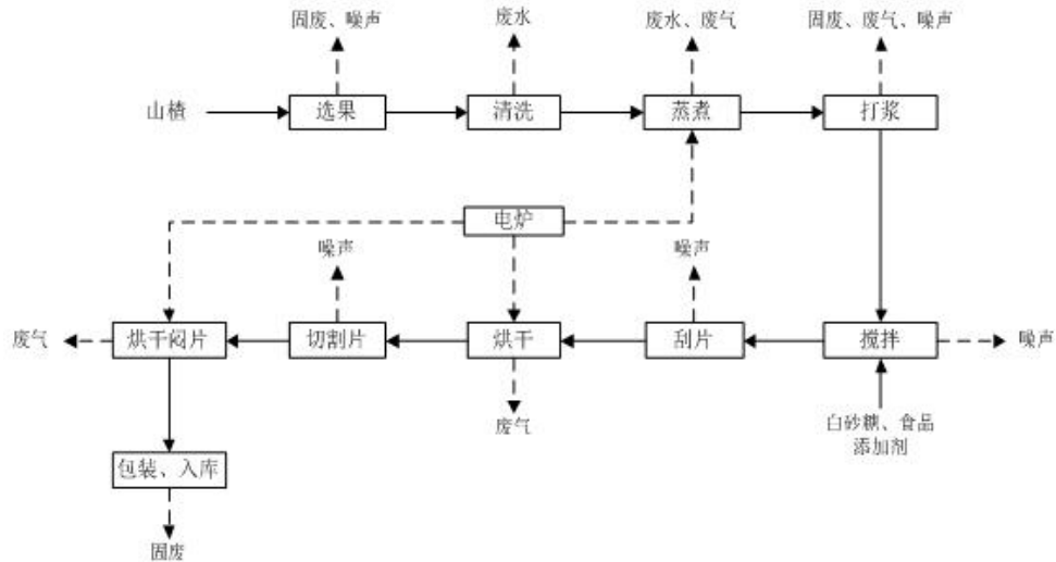
图 1 工艺流程及产污环节示意图
