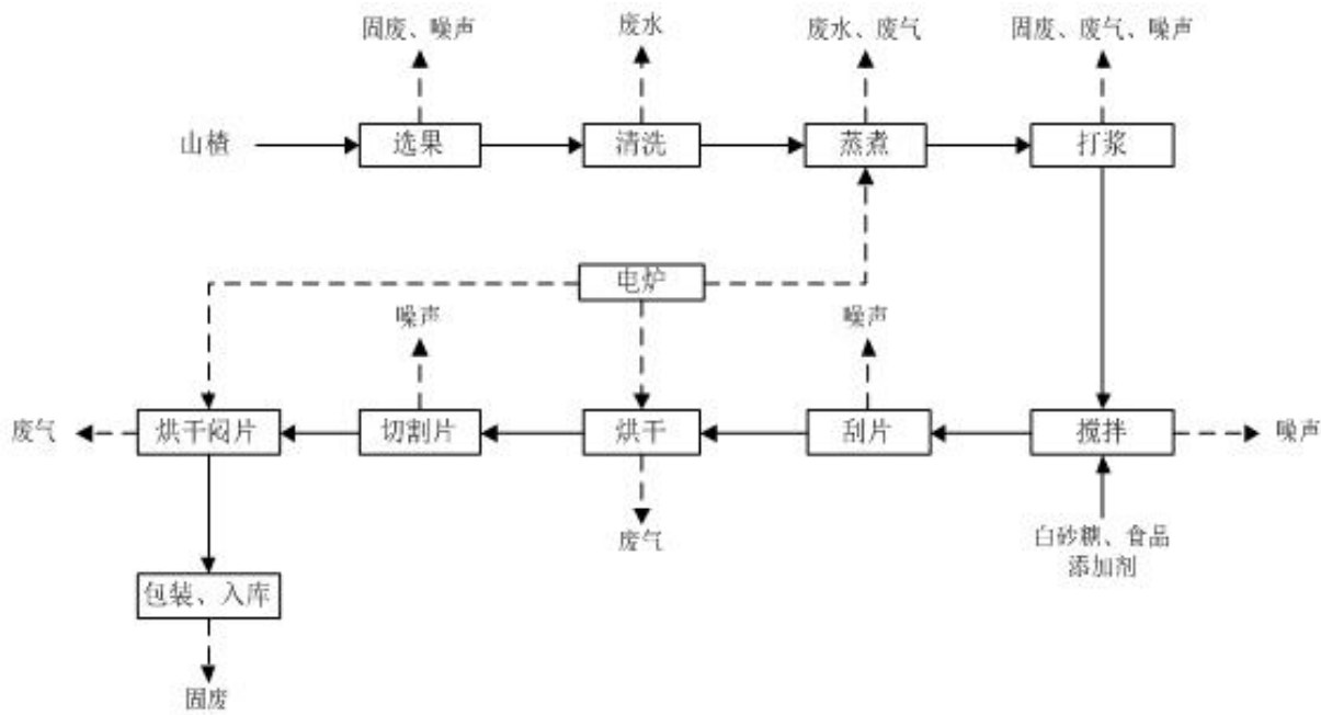
图 2.3-1 工艺流程及产污环节示意图
