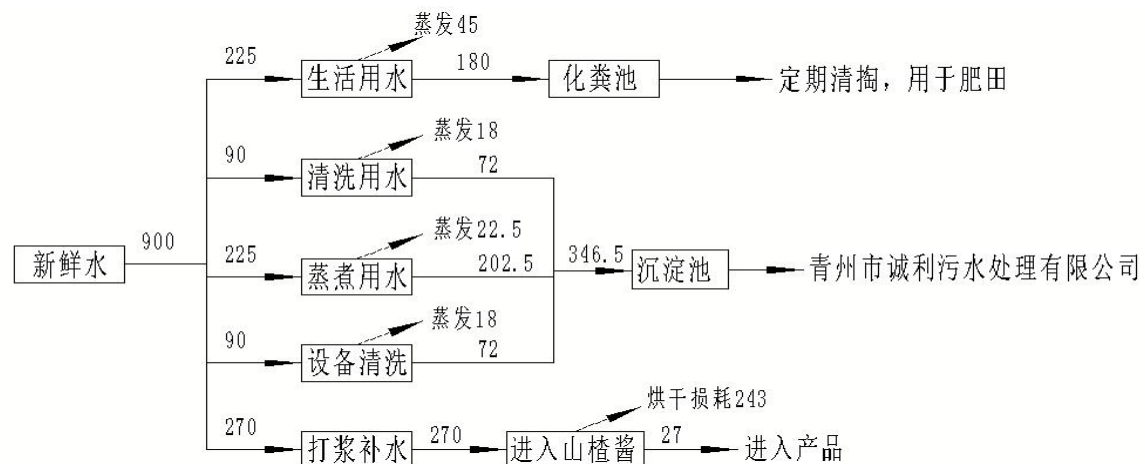
图 2.2-2 项目水量平衡图
