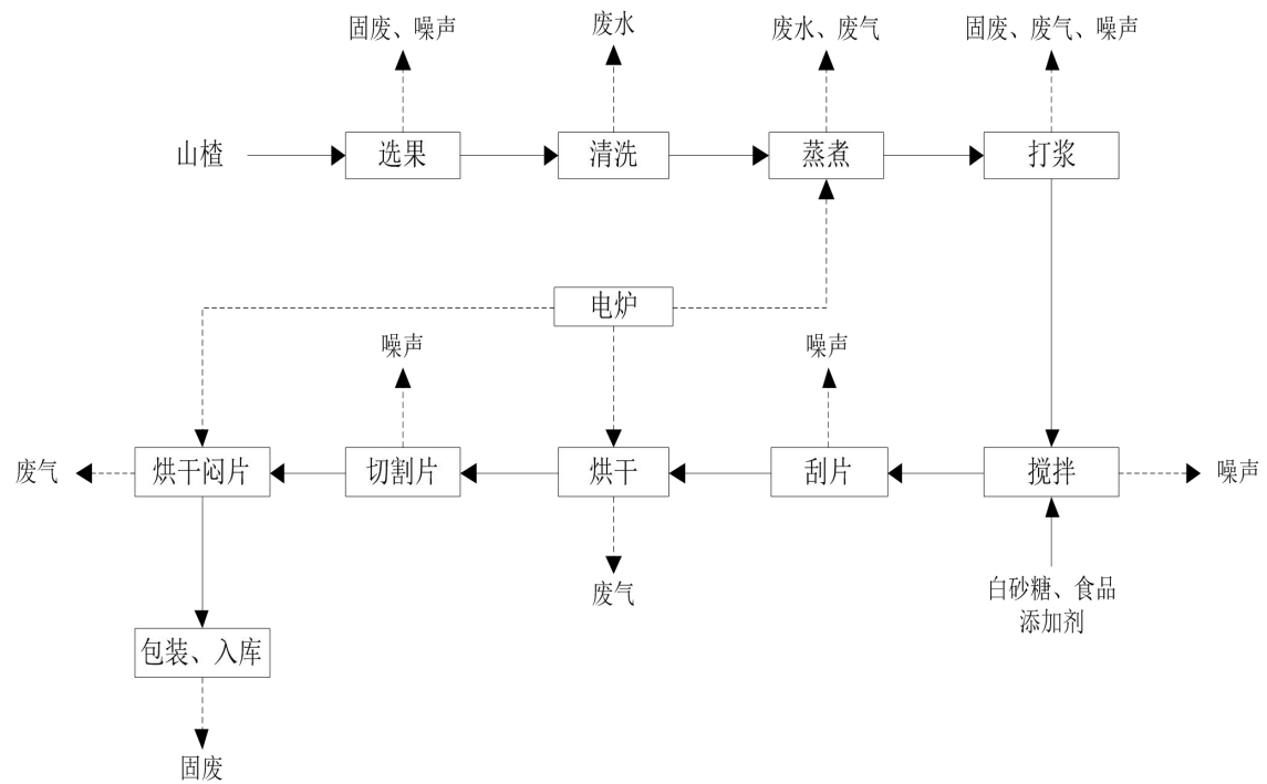
图 2.3-1 工艺流程及产污环节示意图
