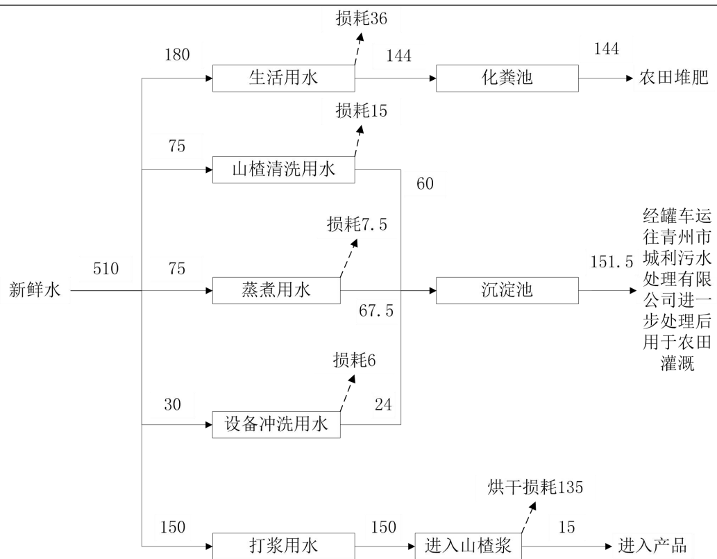
图 2.2-2 项目水量平衡图 单位：m³/a
