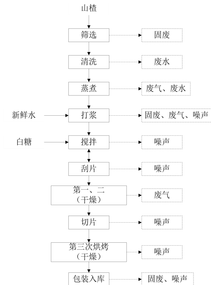
图 1 工艺流程及产污环节示意图
