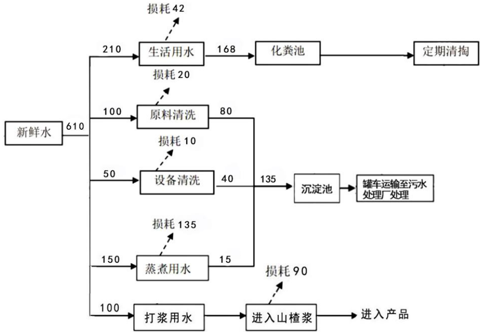
图 2.2-2 项目水量平衡图 单位：m³/a
