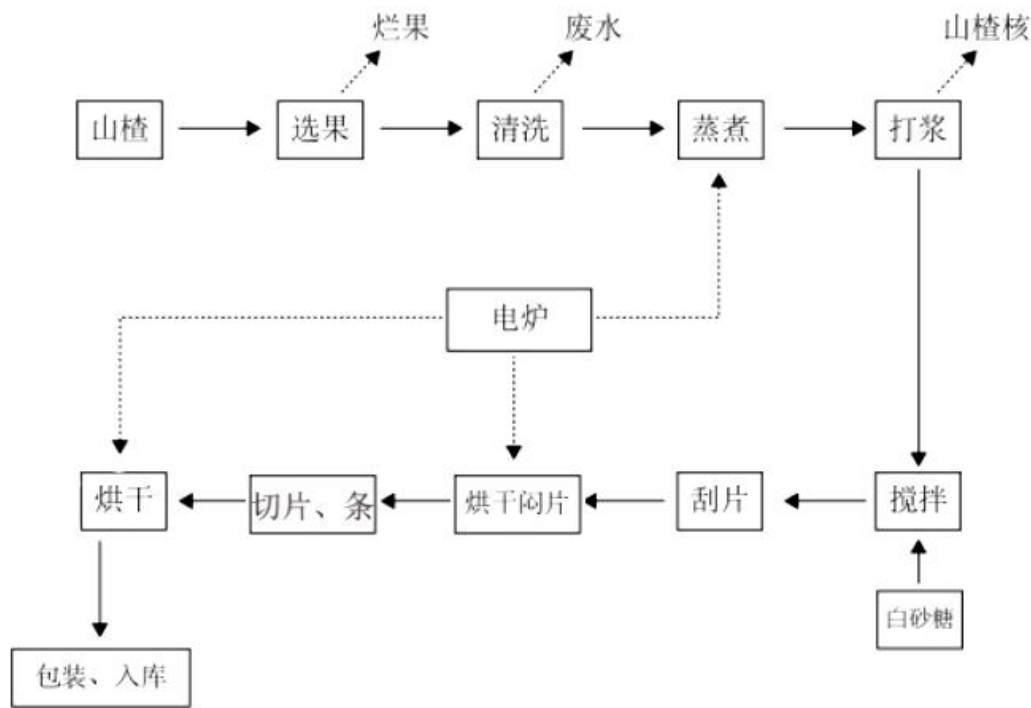
图 2.3-1 工艺流程及产污环节示意图
