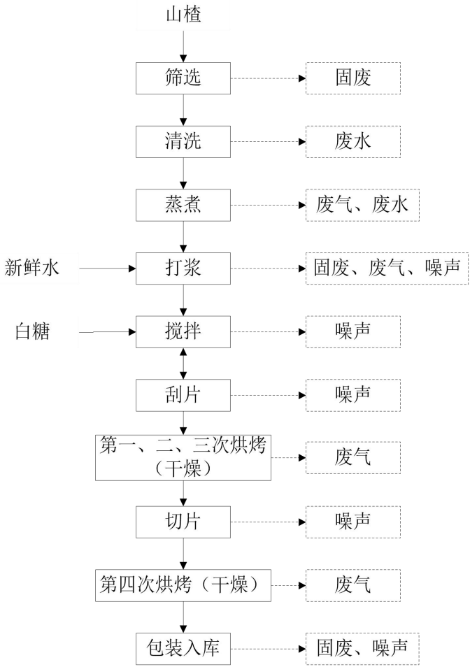
图 2.3-1 工艺流程及产污环节示意图
