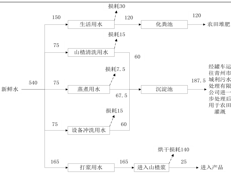
图 2.2-2 项目水量平衡图 单位：m³/a
