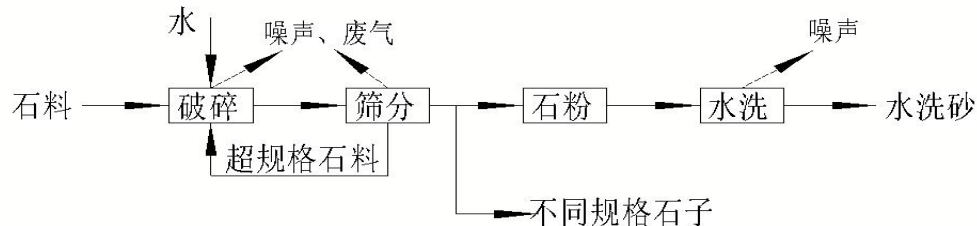
图 1 石子、水洗砂生产工艺流程及产污环节图
