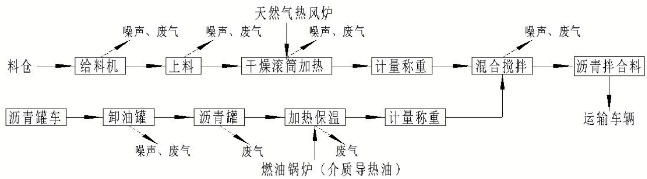
图 2 沥青拌合料生产工艺流程及产污环节图
