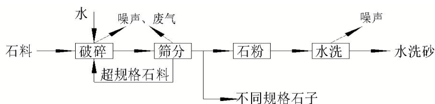
图 2.3-1 石子、水洗砂生产工艺流程及产污环节图
