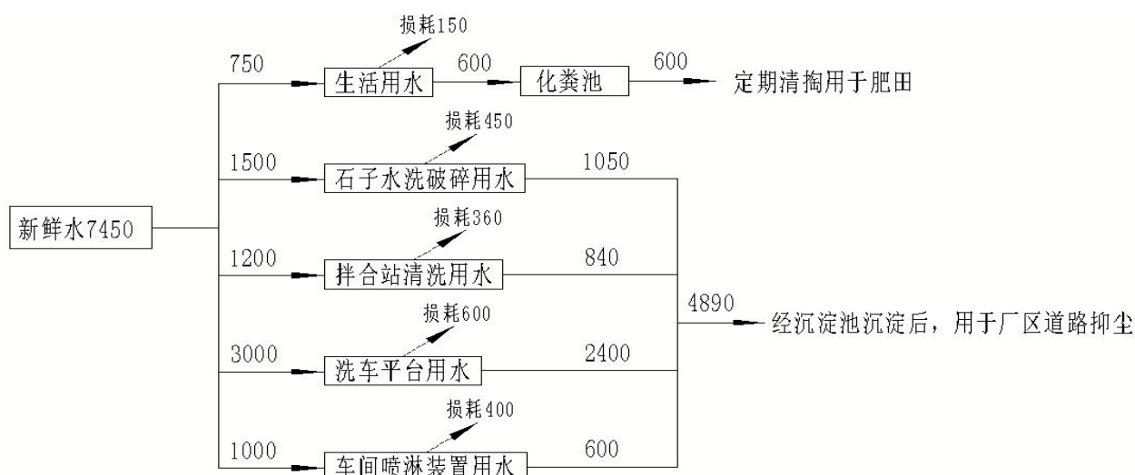
图 2.2-1 项目水平衡图 单位：m³/a
