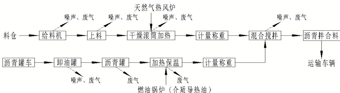
图 2.3-2 沥青拌合料生产工艺流程及产污环节图
