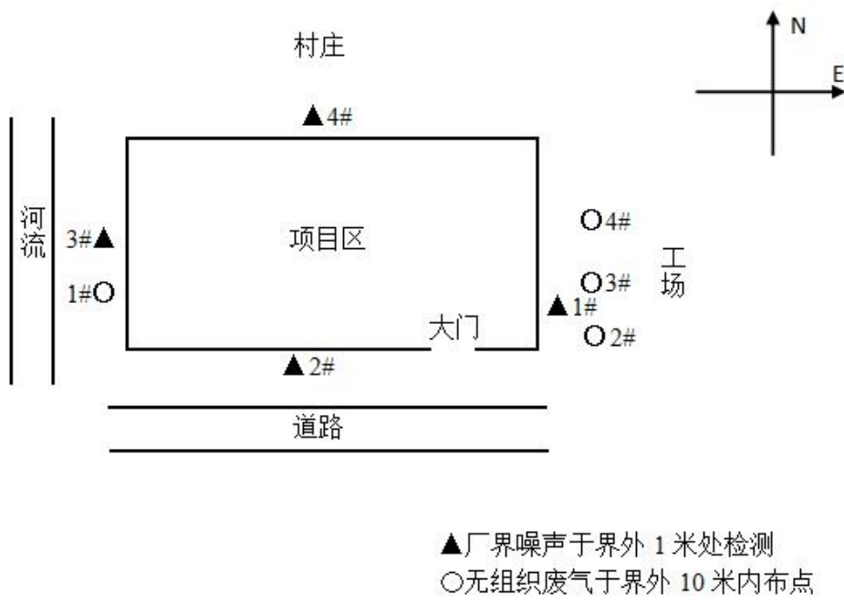
图 6-1 废气和噪声检测点位图
