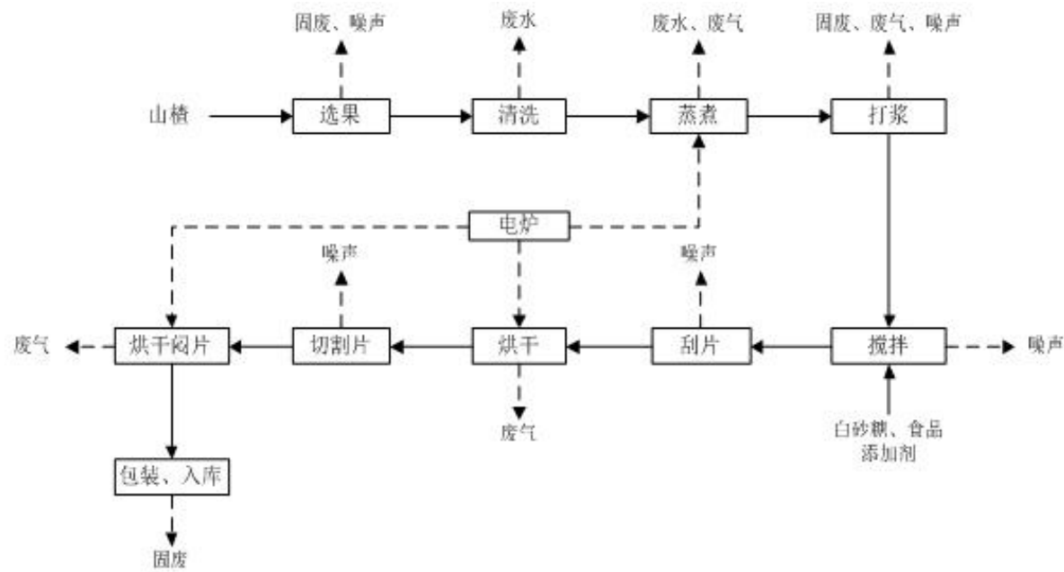
图 2.3-1 工艺流程及产污环节示意图
