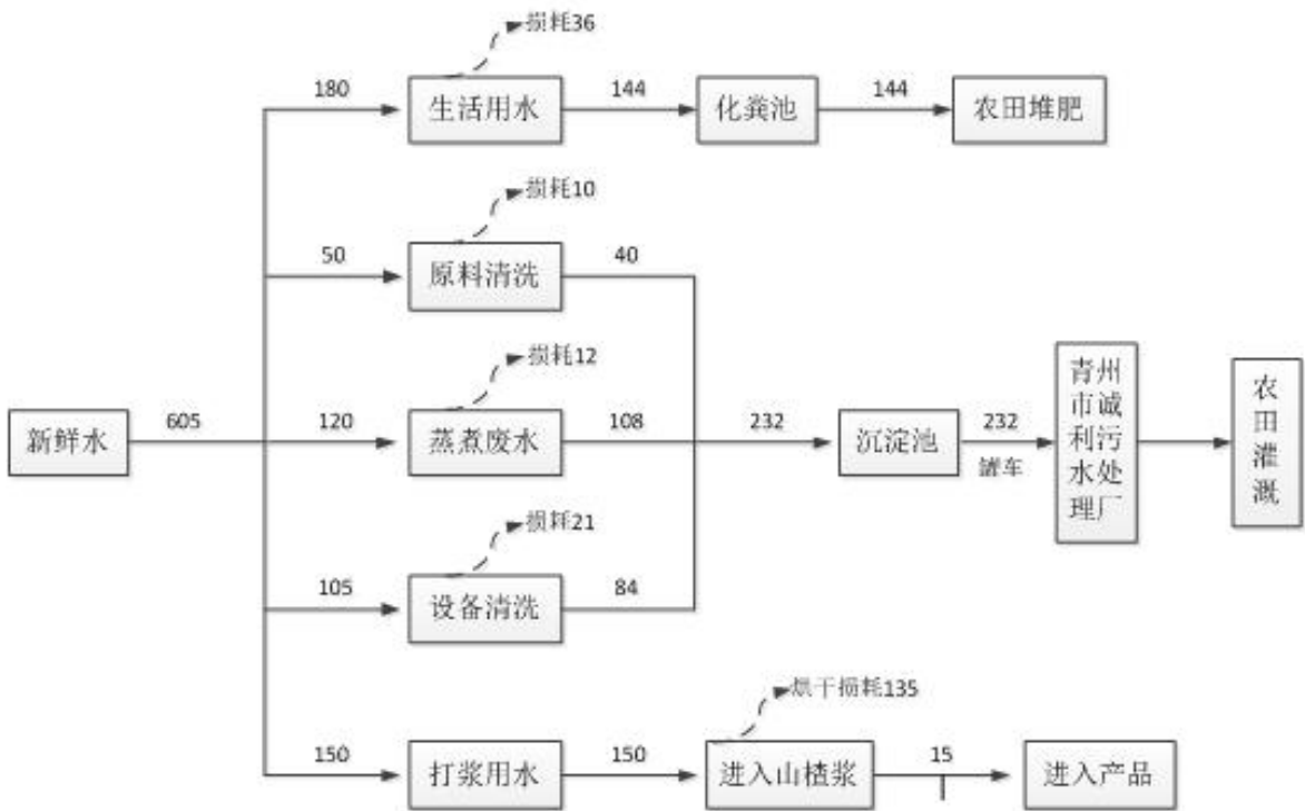
图 2.2-2 项目水量平衡图 单位：m 3 /a
