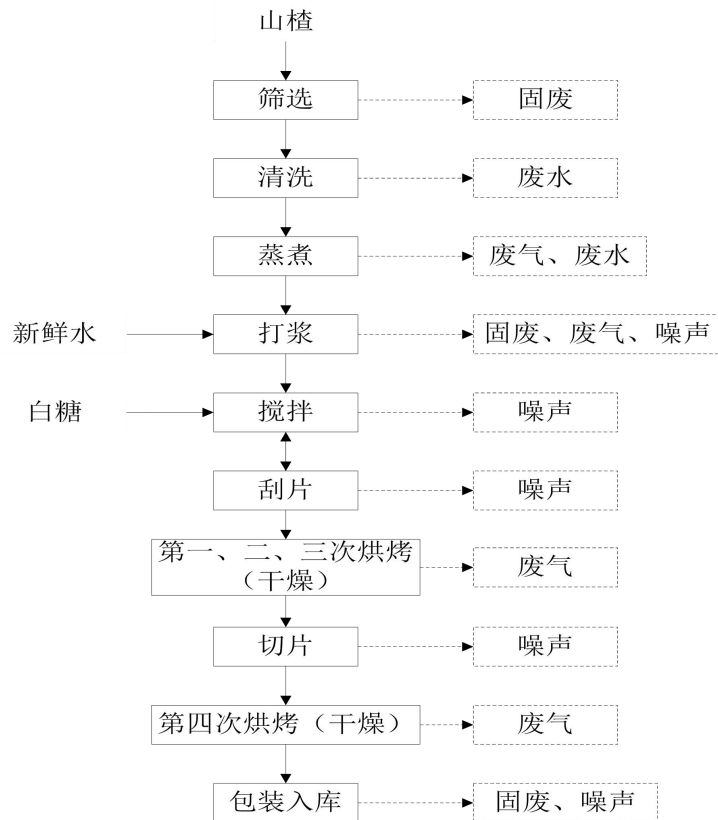
图 2.3-1 山楂片生产工艺流程及产污环节图
