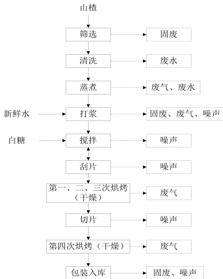
图 1 生产工艺流程及产污环节图
