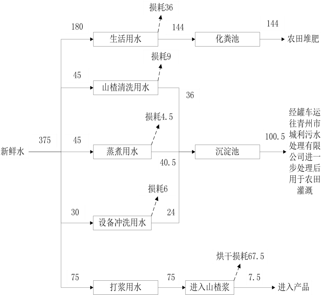
图 2.2-2 项目水量平衡图 单位：m³/a
